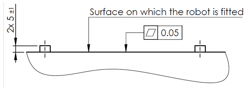
1.2: Montageplatte für Roboterbasis
